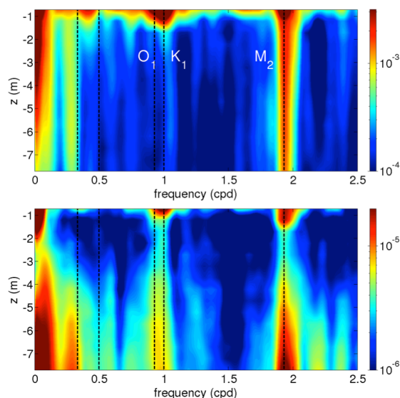
図-4 ADCP 流速データに対する周波数スペクトル解析結果（カラー：対数スケール，単位： \text{m}^2\text{s}^{-1} ）。（上）東向き水平流速，（下）鉛直上向き流速。縦軸：平均海面 z=0 を基準とした鉛直上向き座標，横軸：周波数（cycle/day）（図-5,6 も同様）。
