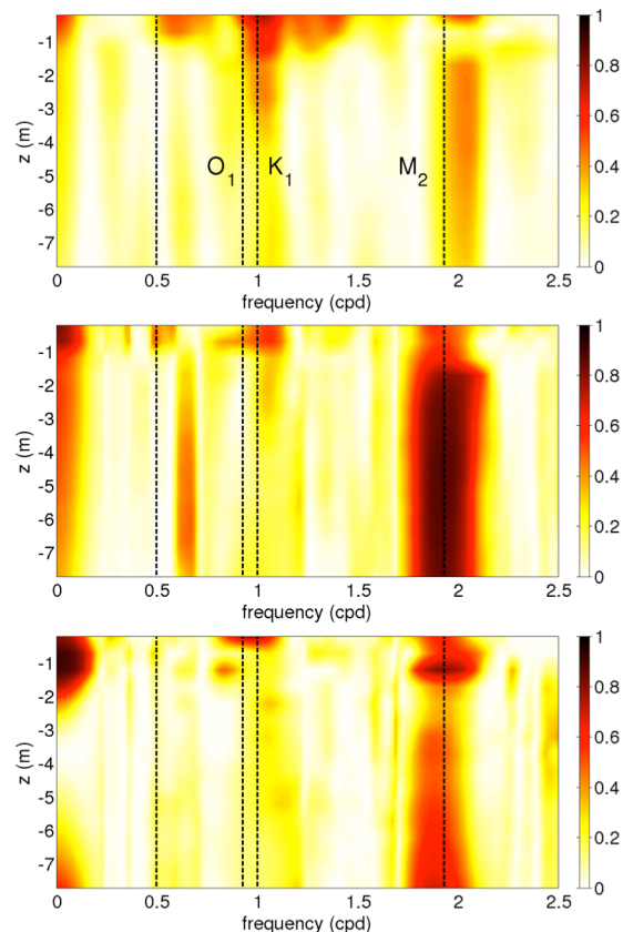
図-5 流速と外力（風速，水位）とのクロススペクトル解析結果。カラー：コヒーレンス（無次元）の鉛直分布。上から順に，東向き風速と東向き流速，水位と東向き流速，水位と鉛直流速のコヒーレンス水深分布。
