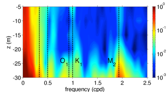
図-6 水温に対する周波数パワースペクトル密度の鉛直分布。単位は ^{\circ}\text{C}^2\text{s} 。図-4,5 とは水深レンジが異なる点に注意。
