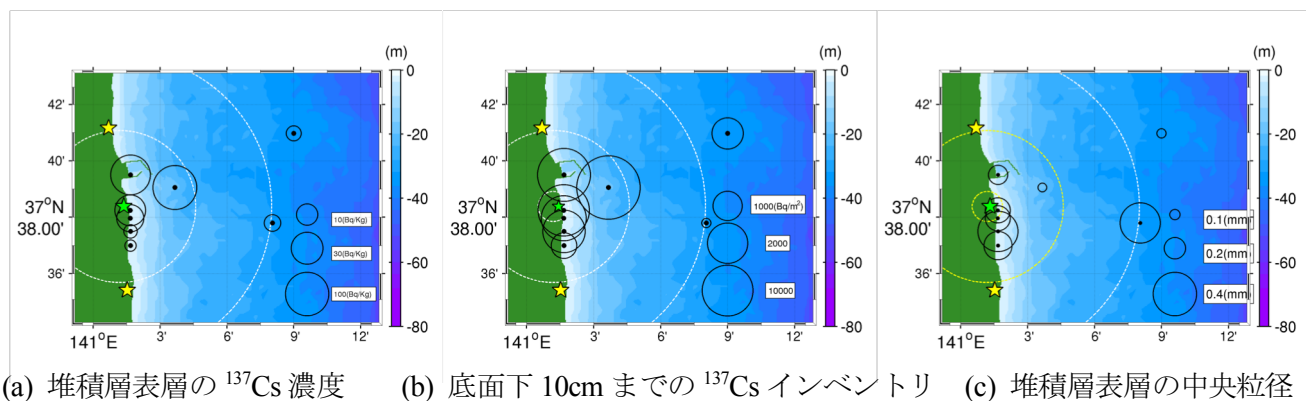
図-2 海底堆積層コアサンプリング結果。円の大きさは各項目(a)~(c)の値に対応。黒丸：観測地点。
